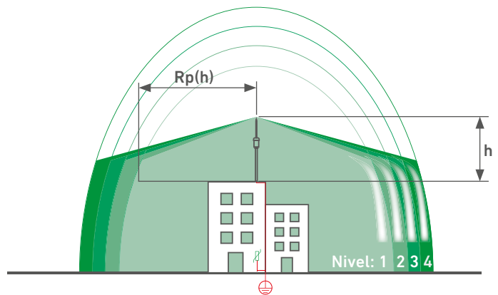
Radio de protección [m] según la norma NF C 17-102:2011 / UNE 21186:2011 / CTE-sección SU8
