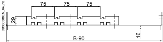
NSYBHS500
