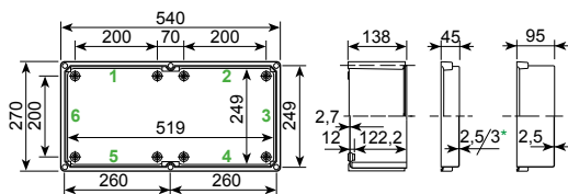
NSYPLS●●●2754●G
