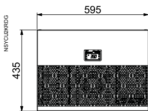
NSYCU2K RDG / NSYCU2K3P4RDG
