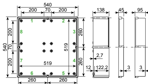
NSYPLS●●●3672●G
