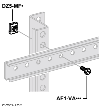
DZ5MF6
