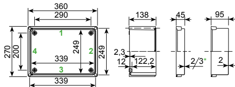
NSYPLS●●●2736●G
