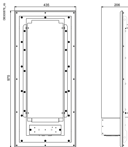
NSYPTDS5
