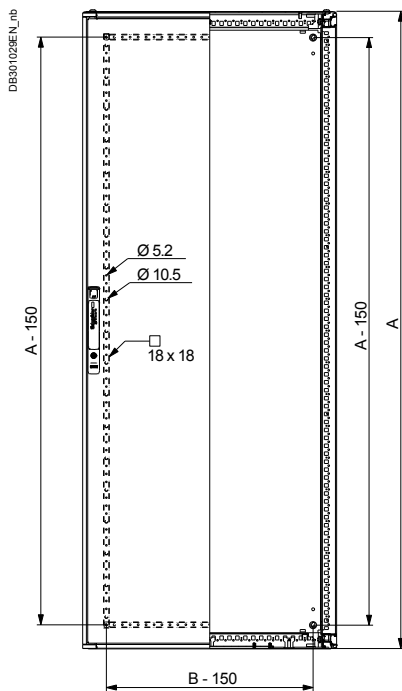
Spacial SFHF
