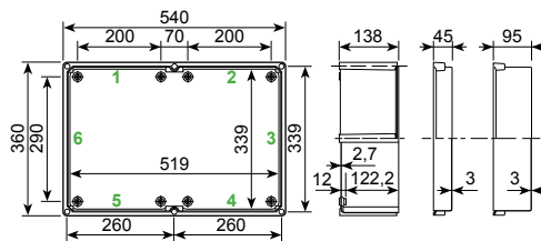
NSYPLS●●●5454●G
