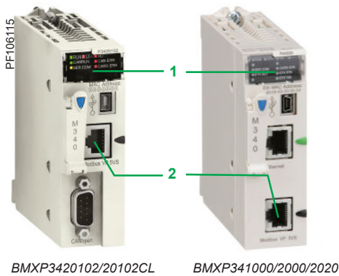
BMXP3420102/20102CL
