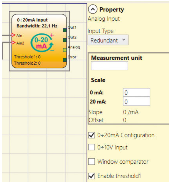
Analogue inputs configuration parameters
