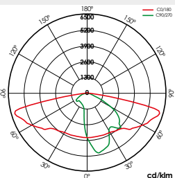
VA01L0M (≤900mA)
