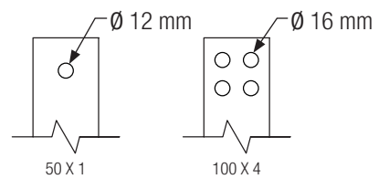
Conexión pletina
