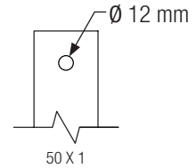
Conexión pletina
