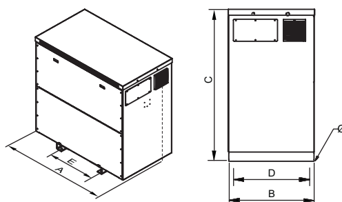
Desde 500 kVA
