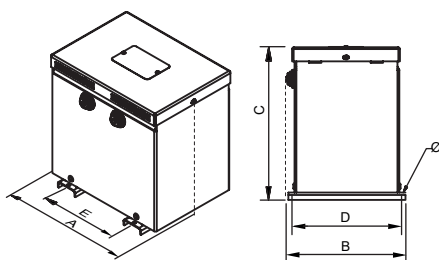
Hasta 1,6 kVA
