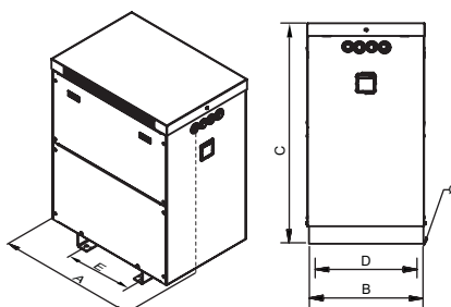
Desde 80 kVA
