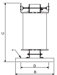
Desde 63 kVA
