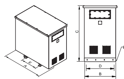
TTUZ IP54
