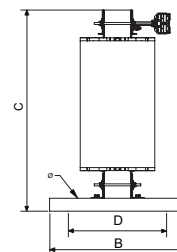
Desde 80 kVA
