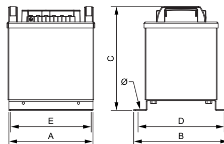
Desde QAU3150
