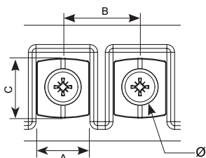
Borne M5
