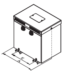
Hasta 3,15 kVA
