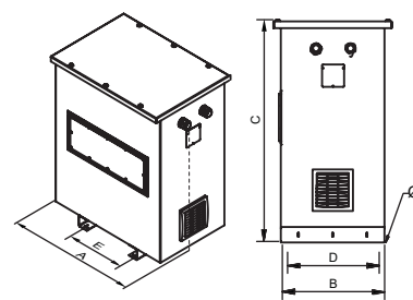
Desde 40 kVA
