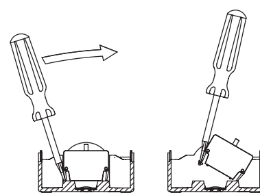
Soltar el bloque de contactos del fondo de la caja
