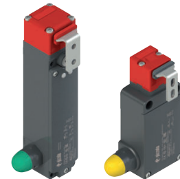
Indicación de una puerta desbloqueada
