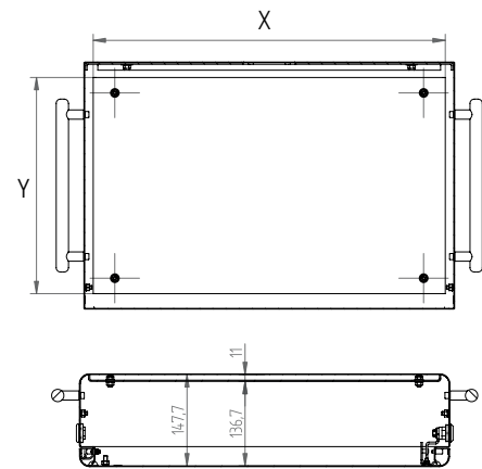
ESPACIO ÚTIL DENTRO DE LA CAJA DE MANDO CON Y SIN PLACA DE MONTAJE
