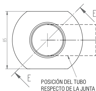
GF48: PARA TUBO Ø 48
