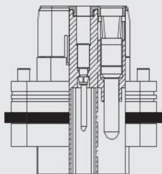
CQM 04/2 / CQM 04/2B
