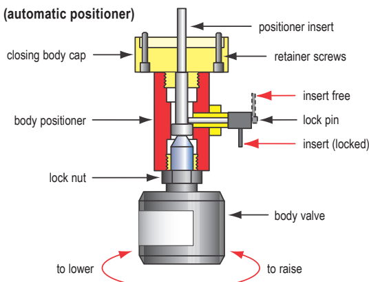
Fig. B (automatic positioner)
