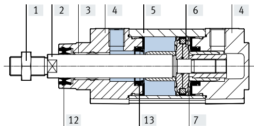
Vista en sección – tipo básico
